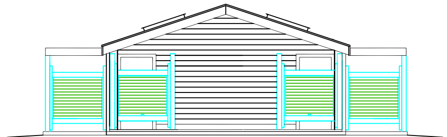
END ELEVATION
